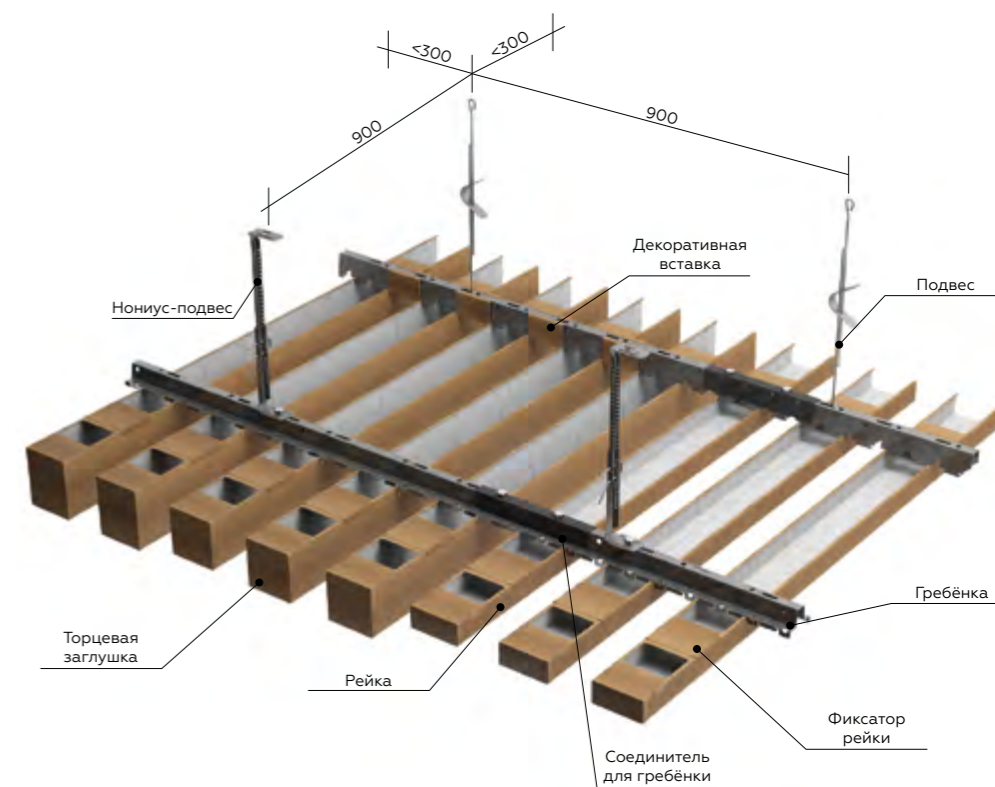
Декоративная вставка гребёнки ВТ-4-50
