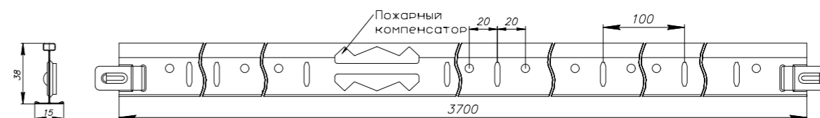
Профиль несущий основной 15/29 L=3700
