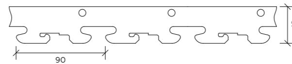
Гребёнка BT 3-90
