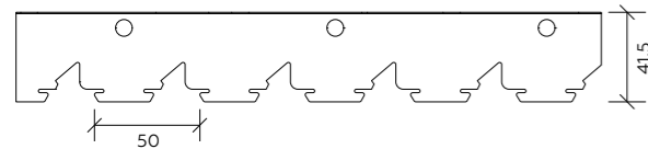
Гребёнка BT 12-50
