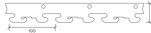
Гребёнка BT 3-100
