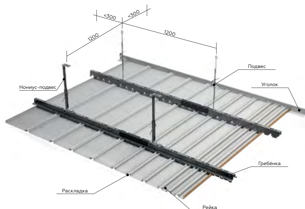
Рейка
