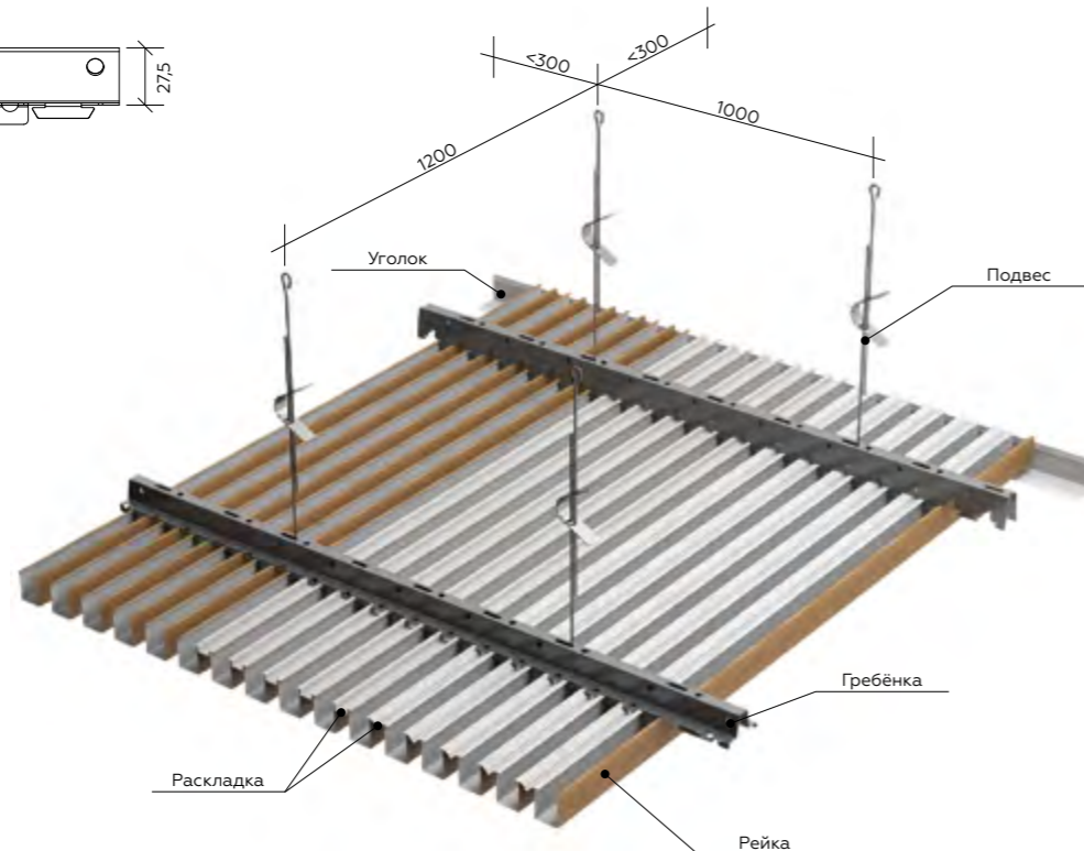
Гребёнка BT 12-50
