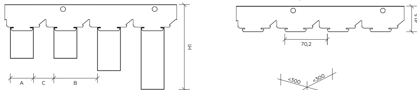
Гребёнка ВТ 4-70
