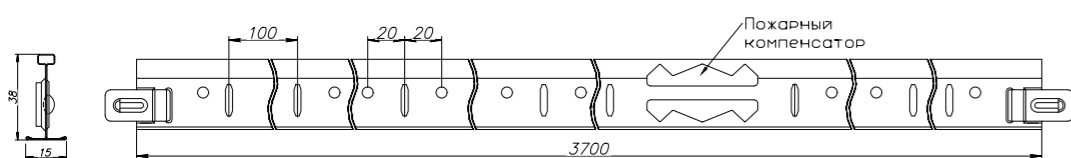
Профиль несущий основной 15/38 L=3700
