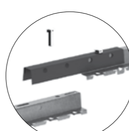
Соед. элемент для гребёнки BT-12-50
