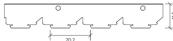
Гребёнка ВТ 4-70
