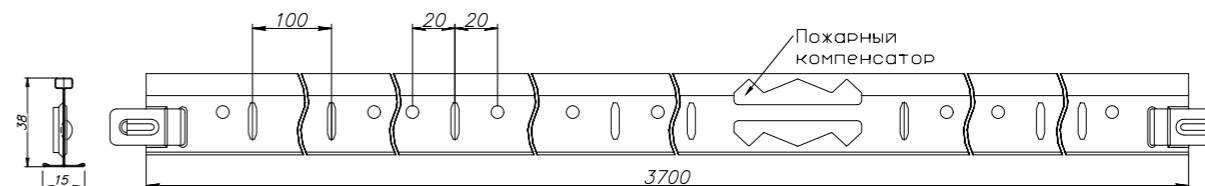
Профиль несущий основной 15/38 L=3700
