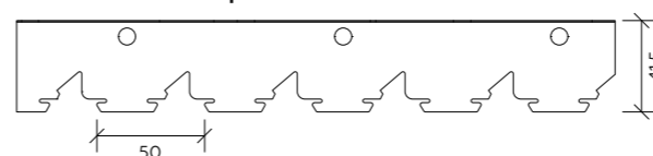
Гребёнка ВТ 4-50
