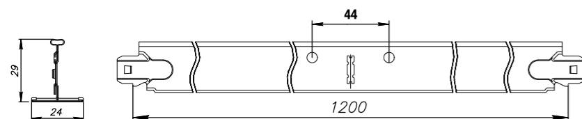
Профиль несущий вспомогательный 24/29 L=1200
