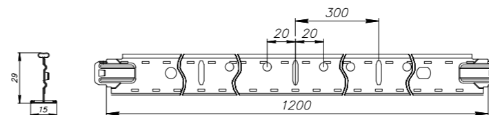
Профиль несущий вспомогательный 15/29 L=1200
