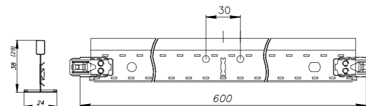
Профиль несущий вспомогательный 24/29, 24/38** L=1200
