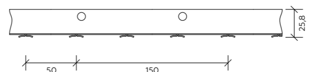
Стык реек
