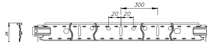
Профиль несущий основной 15/38 L=3700
