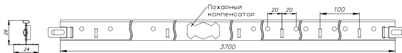
Профиль несущий основной 24/29 L=3700
