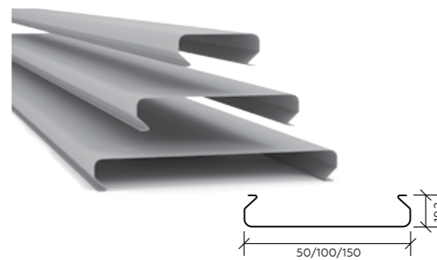
Гребёнка BT-8
