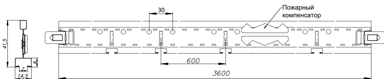
Профиль несущий основной 14,5/41,5 L=3600
