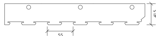
Гребёнка ВТ 19
